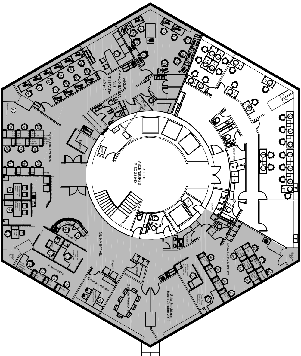
PLANTA EXISTENTE PISO 23
